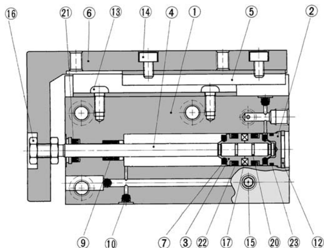
MXU10 (ø10)
