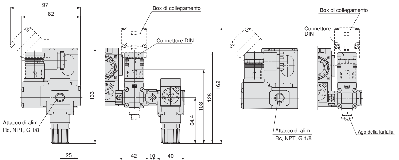
Con regolatore ed elettrovalvola a 2 vie
