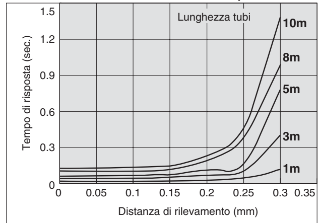
Lunghezza tubi – Tempo di risposta
