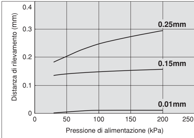
Ugello di rilevamento: \varnothing 1.0 Tubo di rilevamento: \varnothing 6 \times \varnothing 4 tubi 5m
