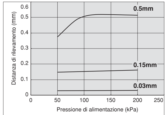
Ugello di rilevamento: \varnothing 1.5 Tubo di rilevamento: \varnothing 6 \times \varnothing 4 tubi 5m
