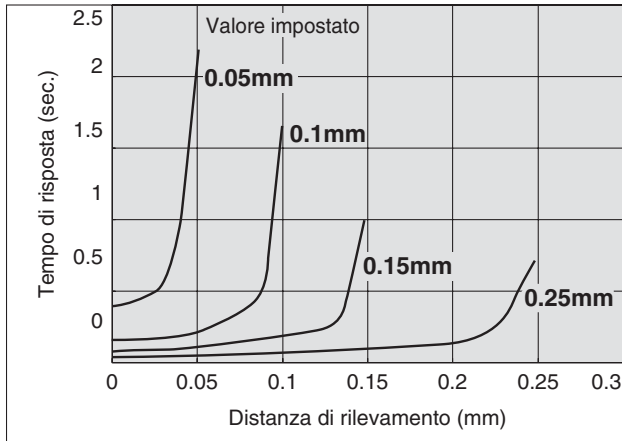
Distanza di rilevamento – Specifiche tempo di risposta
