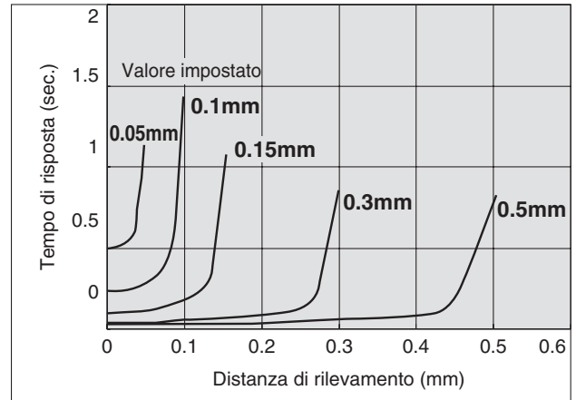
Distanza di rilevamento – Specifiche tempo di risposta
