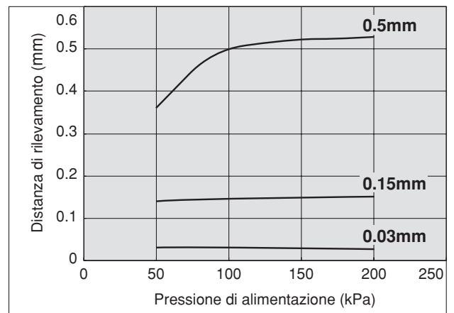
Ugello di rilevamento: \varnothing 2.0 Tubo di rilevamento: \varnothing 6 \times \varnothing 4 tubi 5m
