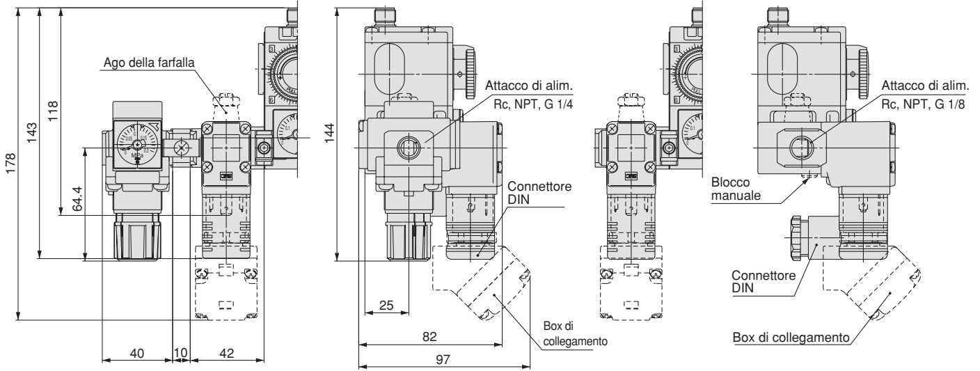
Con regolatore ed elettrovalvola a 2 vie
