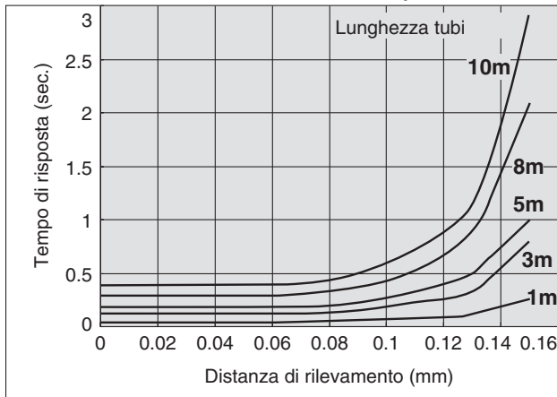
Lunghezza tubi – Tempo di risposta
